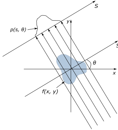
Fig. 4. Basic Radon Transform scenario.
